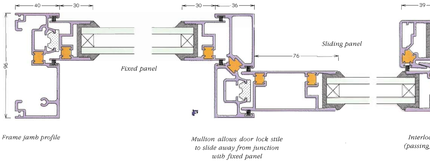
Frame jamb profile
